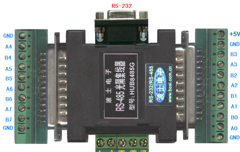
图为波仕新一代 HUB8485G
